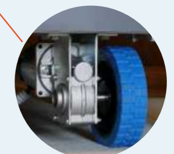
Motore elettrico a lunga durata con ruota motorizzata integrata Ø150mm
