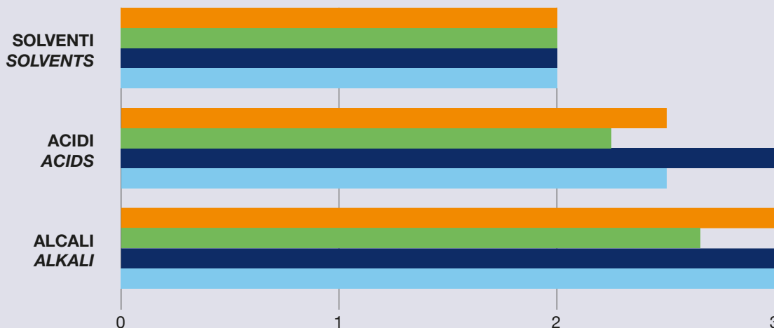
LIVELLO DI RESISTENZA ALLA PERMEAZIONE (RISULTATO MEDIO) - LEVEL OF RESISTANCE TO PERMEATION (AVERAGE)
